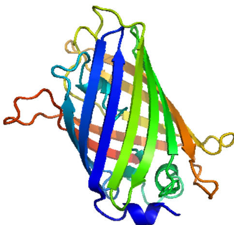
Рис. 1. Тривимірна структура (стрічкова діаграма) зеленого флуоресцентного білка (GFP). Білок представляє собою типову бета-складчасту структуру з 11 поворотів первинної послідовності у формі «бочечки» чи «циліндра», всередині якого є флуорофор*. (*джерело зображення — Банк даних білків (Protein Data Bank, PDB))
